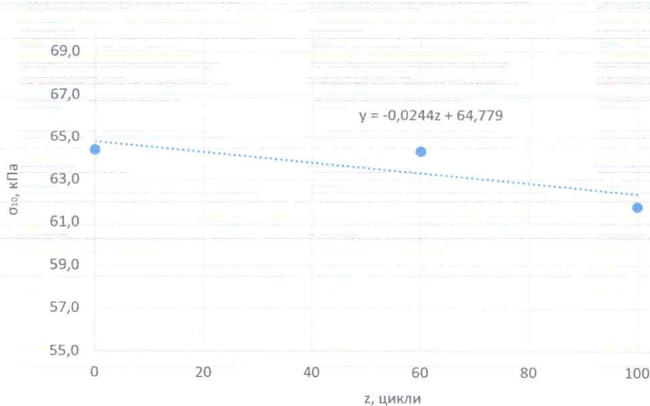
Рисунок 7 – Залежність міцності на стиск при 10% деформації від циклічних впливів зразків № 70/23 теплоізоляційного матеріалу марки «ТЕХНОРУФ ПРОФ»
