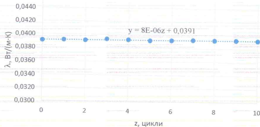
Рисунок 5 – Залежність теплопровідності від циклічних впливів
